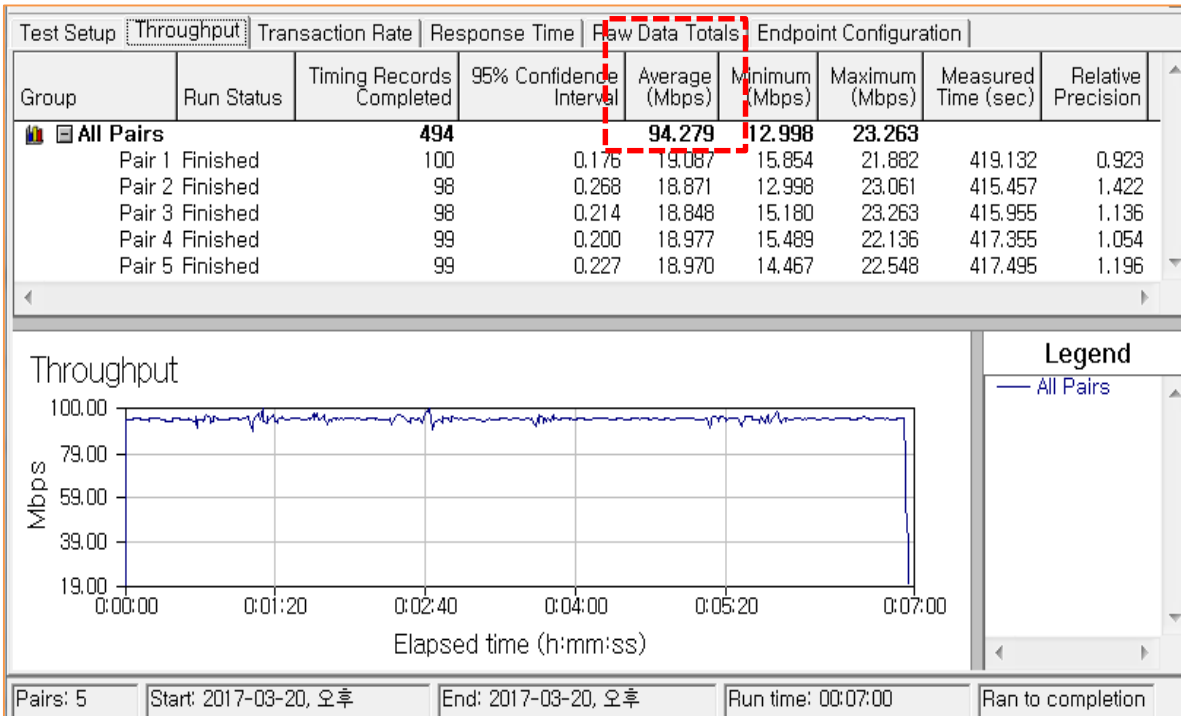
1.3Km 지점 throughput 측정
